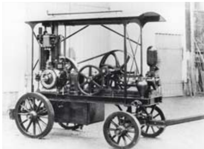
Erste benzinmotorgetriebene Feuerspritze der Welt: Daimler 1-Zylinder mit einem PS aus dem Jahr 1888.
